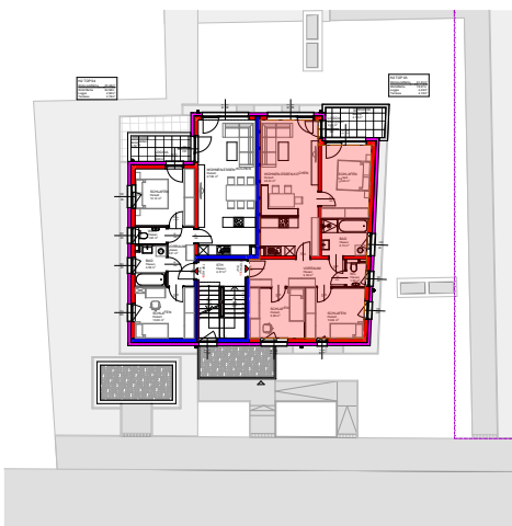
ÜBERSICHT LAGEPLAN 1:500
