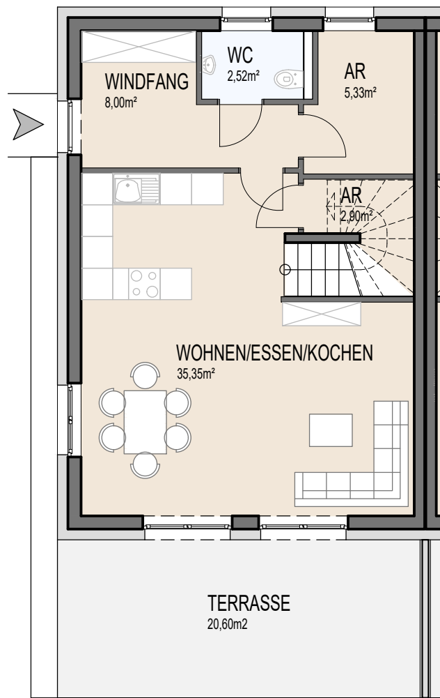
ERDGESCHOSS
