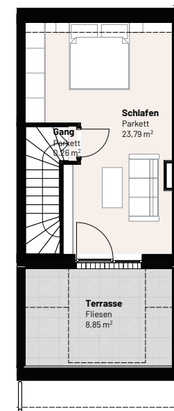
DACHGESCHOSS | M 1:100
