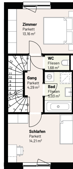
OBERGESCHOSS | M 1:100
