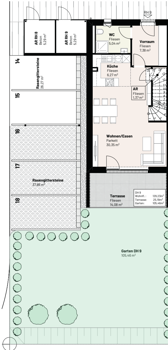
ERDGESCHOSS | M 1:100
