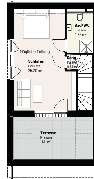
DACHGESCHOSS | M 1:100
